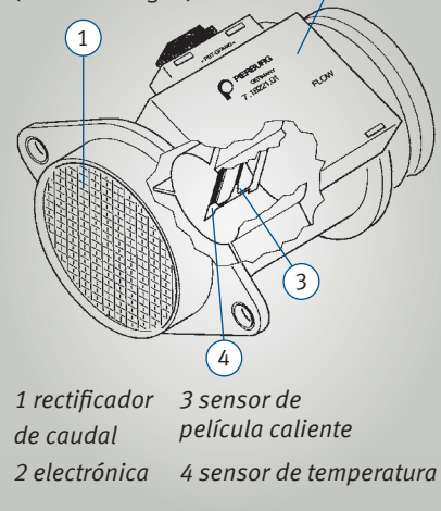
LMS de película caliente (modelo antiguo)
