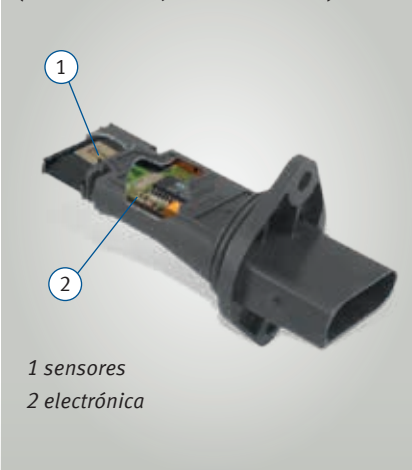
LMS de película caliente (modelo nuevo, corte en sección)
